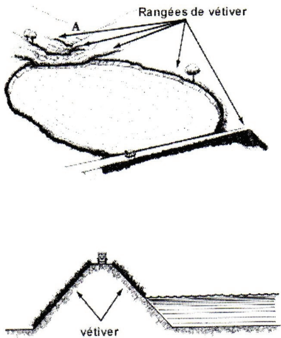
Figure 47. Protection des barrages
