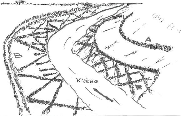
Figure 24. Protection des berges en quinconce
