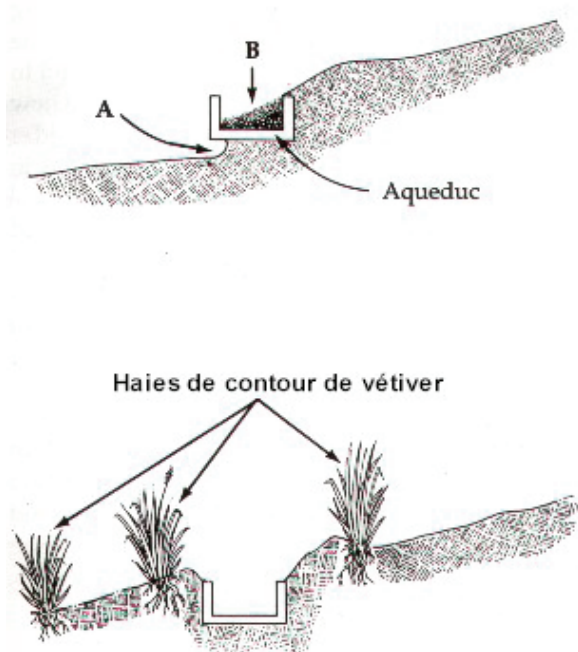
Figure 36. Canaux d'irrigation en dur sur collines
